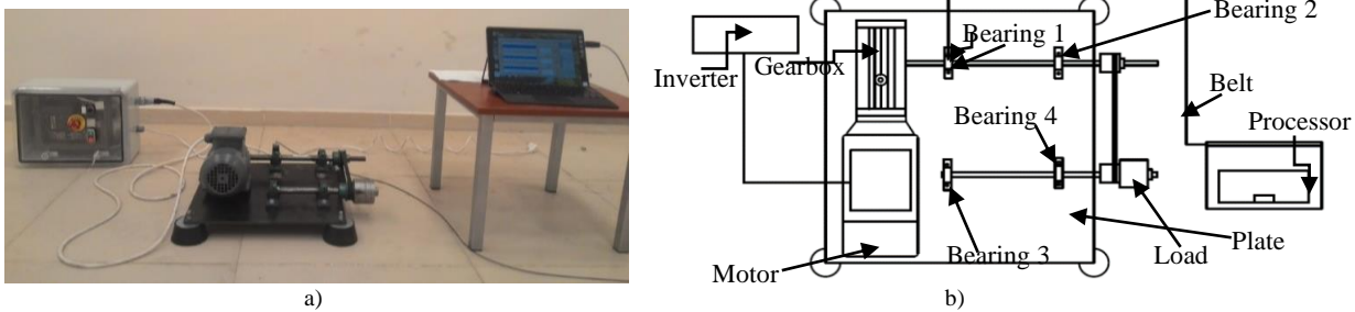
Fig. 1 Test setup: a) Actual view, b) Schematic view
