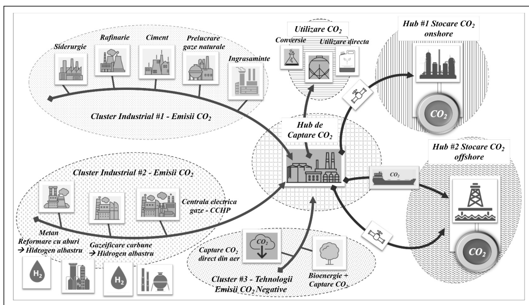
Fig. 14. Model generalizat al conceptului „clean energy hub connected to CO 2 emissions industrial cluster” – „centre de energie curată asociate platformelor industriale cu emisii GES”.
