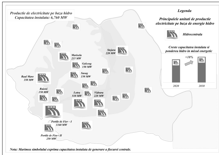
Fig. 9. Principalele hidrocentrale din România – capacități instalate și evoluția ponderii hidro în mix-ul energetic 2020/2030 (sursa datelor primare: Transelectrica, 2020).
