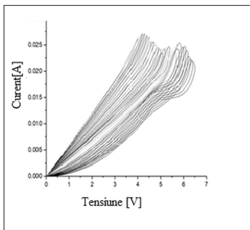
Fig. 1 Caracteristici I-V ale unui memristor pe bază de IGZO
