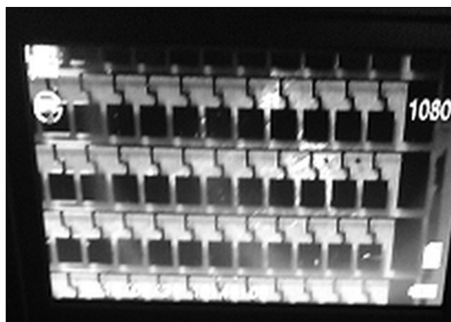
Fig. 3 Matrice de memristoare IGZO realizată pe suport de sticlă
