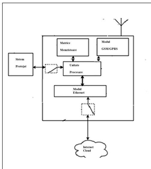
Fig. 6 Schema bloc a sistemului dezvoltat
