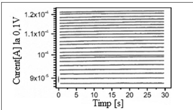
Fig. 5 Diferite stări ale unui memristor citit la 0.1V
