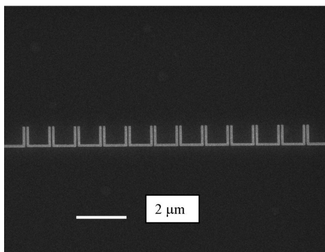
Fig. 2 MoS 2 nanoradio [14]
