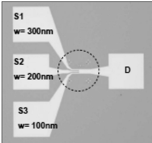
Fig. 6 Tranzistor reconfigurabil grafenă/HfZrO
