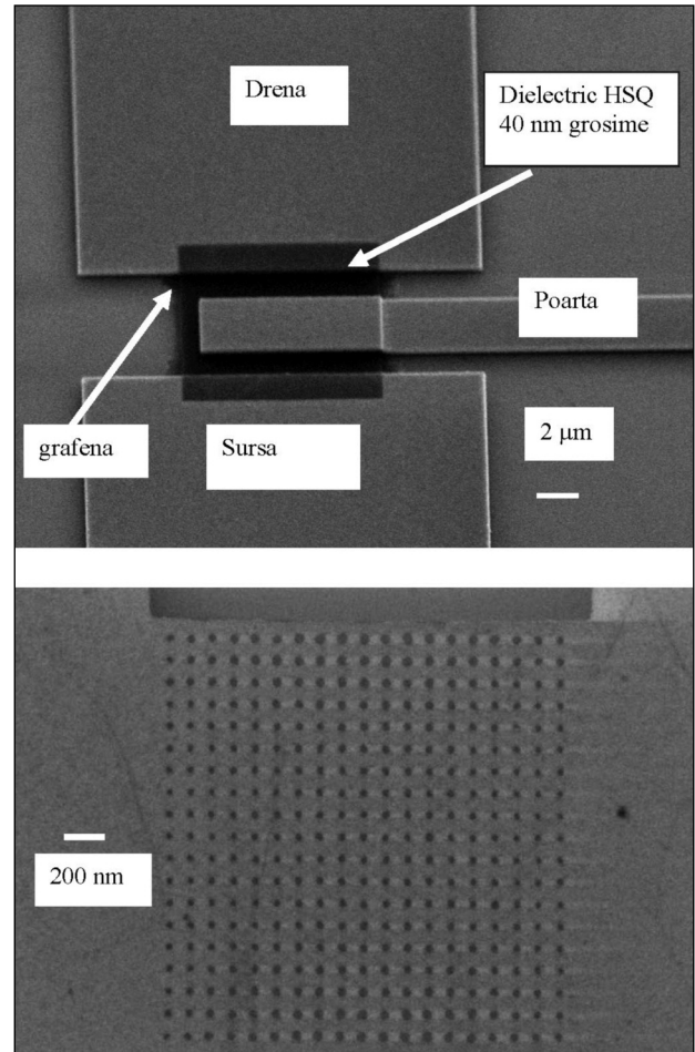
Fig. 5 (a) FET grafenă (b) canal grafenic imprimat cu o structura periodică [15]
