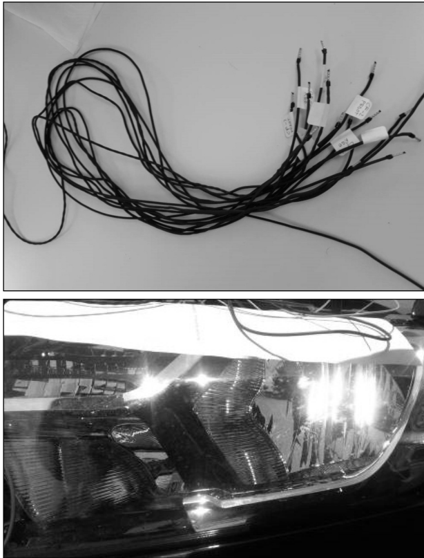
Fig. 4 Cabluri electrice grafenice pentru iluminarea farurilor automobilelor
