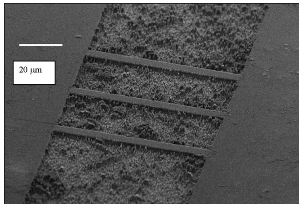
Fig. 1 Trei nanomembrane de GaN care prin efect memristiv imită mecanismele de învățare de tip obișnuință, dezobișnuință, memorare [12]
